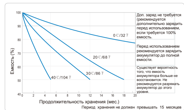
Характеристики саморазряда
