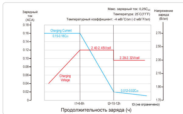
Профиль заряда
