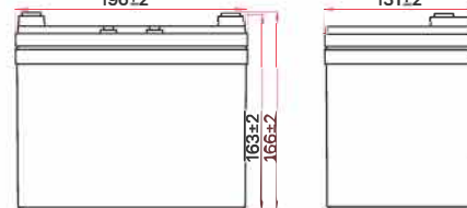
Габаритные размеры, мм
